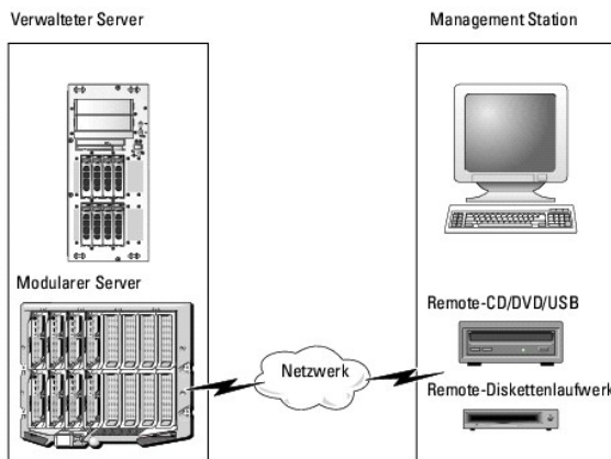
Abbildung 12-1. Gesamte Architektur des virtuellen Datenträgers
